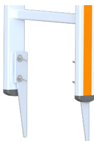
Paire de pointes pivotantes pour sol agricole, fixées
