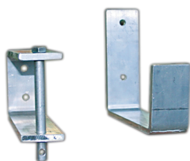
Fixation murale verrouillable, 1 paire, dimension intérieure 240 mm
