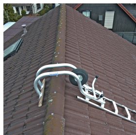
Crochet de faîtage pour échelle de couvreurs
