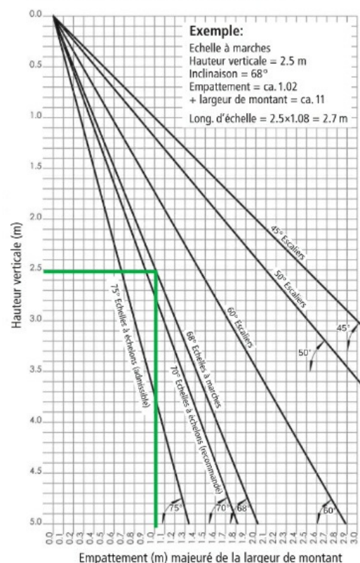
Diagramme pour le calcul de l'empattement
