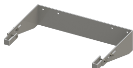
Fixation murale en forme de U, pour échelle à crinoline, ajustable 275-375 mm
