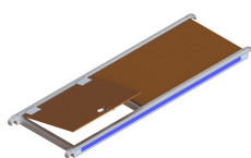
Plateforme de travail 180/60 avec clapet
