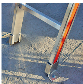
Paire d'équerres de fixation au sol pour échelles à échelons, pour montant du profil 70
