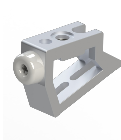
1 paire d'adaptateurs n° 3, largeur du montant 66-100 mm
